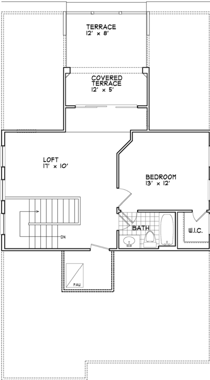
OPTIONAL LOFT LEVEL A: 592 SQ. FT
